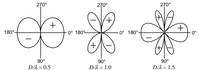
Fig. 3. Polardiagramme für charakteristische Frequenzen
