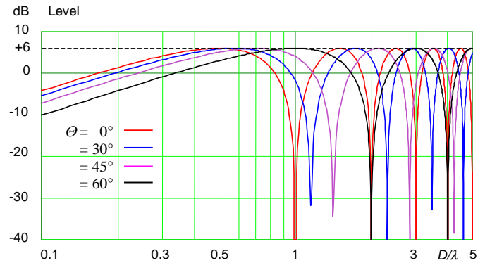
Fig. 2. Betragsfrequenzgang |H(\omega)| als Funktion von D/\lambda für \theta = 0^\circ, 30^\circ, 45^\circ, 60^\circ (von oben nach unten)
