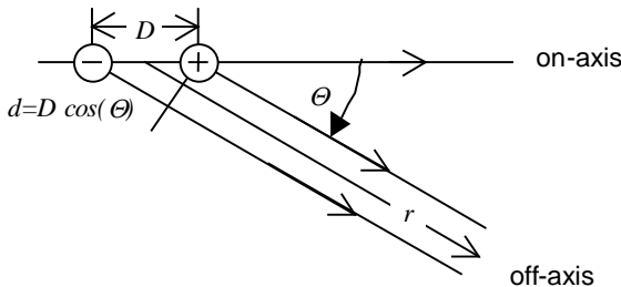
Fig. 1. Schematische Darstellung eines Gradientenstrahlers 1. Ordnung (aus [6])
